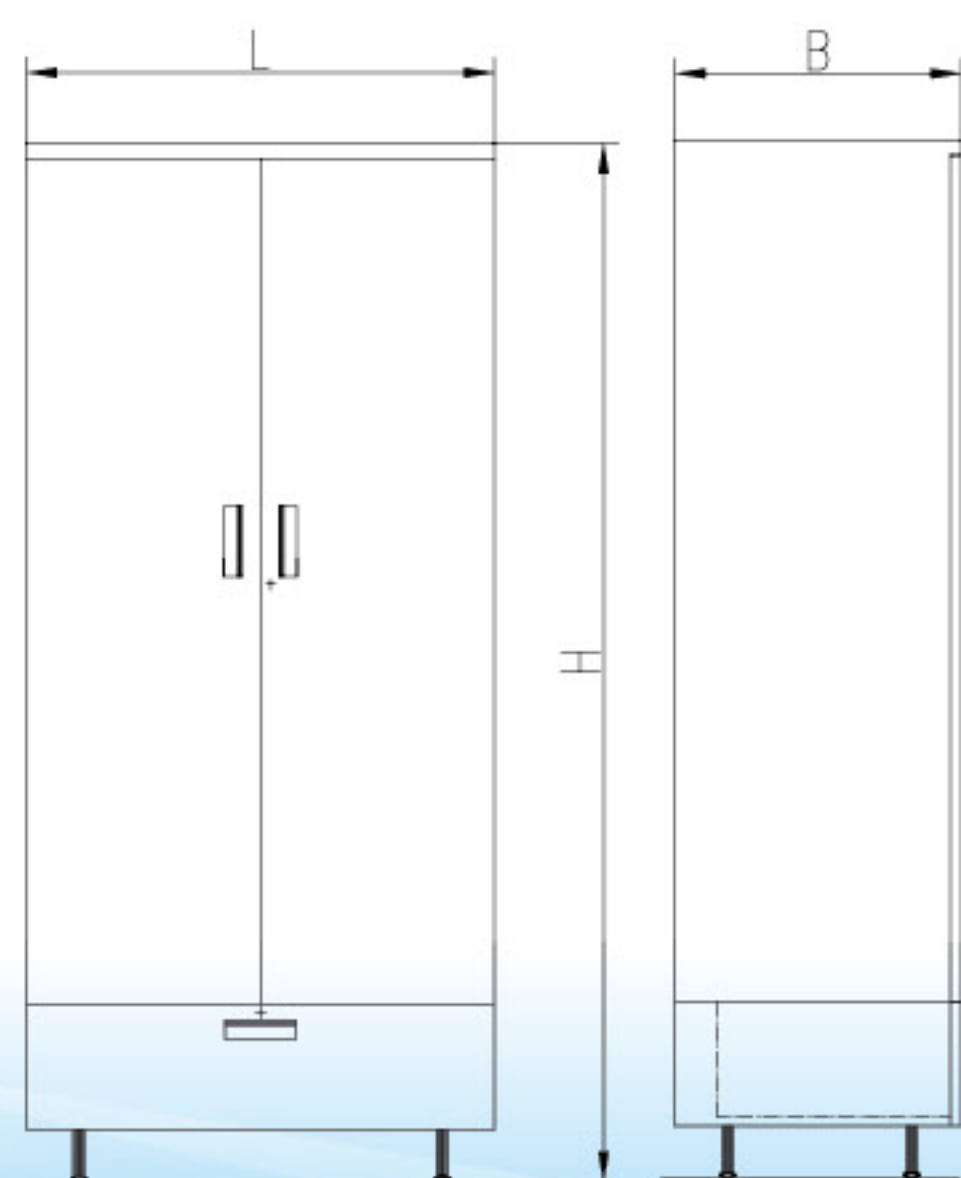
双门衣柜 Double Closet
